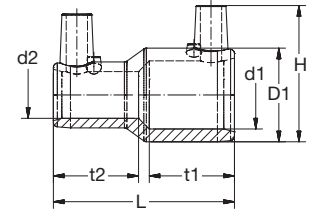
PE100 E-Reduktion SDR11 schwarz 39003 PE100 E-Reducer SDR11 black
