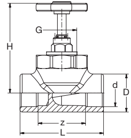
G 8599cB PP-RCT-RG Ventil Geradsitz mit Handrad grün PP-RCT-Bronze Valve straight with hand wheel green
