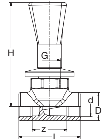
G 8599dB PP-RCT-RG Ventil Geradsitz UP mit Flügelrad + Kappe grün PP-RCT-Bronze Valve straight concealed with winged wheel + cap green
