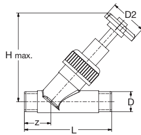
621.300.000 PVC-U Ventil Schrägsitz Runddichtring-PB grau PVC-U Valve angle-seat O-Ring-gasket-PB grey
