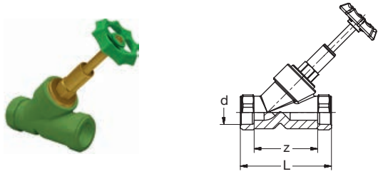
G 8700 PP-R-RG Ventil Schrägsitz mit Metallsitz grün G 8700/1 PP-R-Bronze Valve angle with metal seat green
