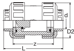
621.360.000 PVC-U Ventil Rückschlag Runddichtring-EPDM grau PVC-U Valve non-return O-Ring-gasket-EPDM grey
