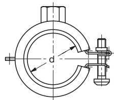
8500 Rohrschelle STANDARD mit Gummieinlage grün Pipe clamp STANDARD with rubber insert green
