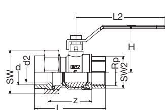
PP-R Ü-Kugelhahn-Ms IG-zyl verschraubt Runddichtring-EPDM grün PP-R Transition-Ball valve Brass female-thread-cyl with union-nuts O-Ring-gasket-EPDM green
