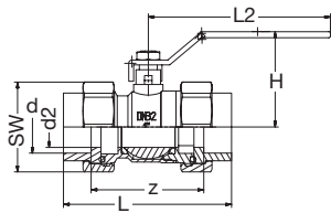
PP-R Kugelhahn-Ms verschraubt Runddichtring-EPDM grün PP-R Ball valve Brass with union-nuts O-Ring-gasket-EPDM green
