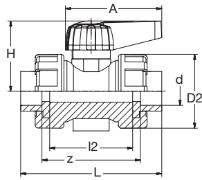
G 8852B PP-R Kugelhahn verschraubt Runddichtring-EPDM 20°C/1.0MPa grün PP-R Ball valve with union-nuts O-Ring-gasket-EPDM 20°C/1.0MPa green
