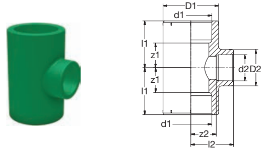
G 8130B red PP-RCT T-Stück 90° red grün PP-RCT Tee 90° red green
