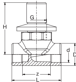
G 8599bB PP-RCT-RG Ventil Geradsitz UP mit Drehgriff grün PP-RCT-Bronze Valve straight concealed with handle bar green
