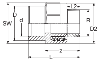
620.91.07 PVC-U-RG Übergang AG-keg grau PVC-U-Bronze Transition male-thread-con grey
