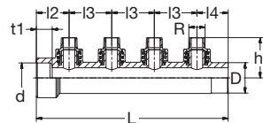
G 8241g PP-R-RG Verteiler AG-keg kaskadierbar grün PP-R-Bronze Manifold male-thread-con cascable green
