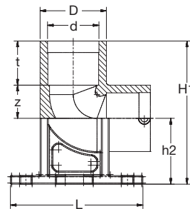
PE100 E-Fußbogen 90° SDR11 schwarz 31103 PE100 E-Duckfoot Elbow 90° SDR11 black
