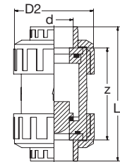
21.10.140 PVC-U Ventil Fuß Runddichtring-EPDM grau PVC-U Valve foot O-Ring-gasket-EPDM grey
