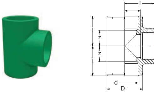
G 8130B PP-RCT T-Stück 90° grün PP-RCT Tee 90° green
