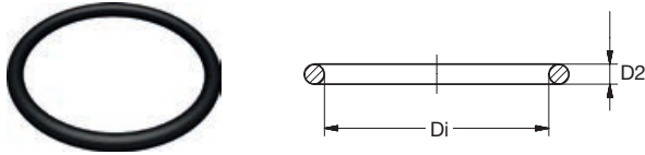
Runddichtring für Bundbuchsen mit O-Ring-Kammer schwarz O-Ring gasket for flange adaptor socket with O-Ring chamber black
