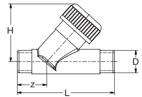
621.303.000 PVC-U Ventil Schrägsitz Rückschlag Runddichtring-EPDM grau PVC-U Valve angle-seat non-return O-Ring-gasket-EPDM grey
