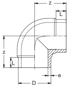
25.10.01.101 PE100 Winkel 90° kurz SDR11 schwarz PE100 Elbow 90° short SDR11 black
