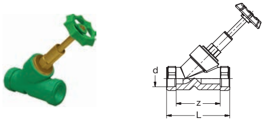
G 8700B PP-RCT-RG Ventil Schrägsitz mit Metallsitz grün G 8700/1B PP-RCT-Bronze Valve angle with metal seat green
