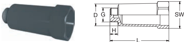
9900 Abpreßzapfen AG-zyl mit NBR-Runddichtring Wall inlet plug male-thread-cyl with NBR-O-Ring gasket
