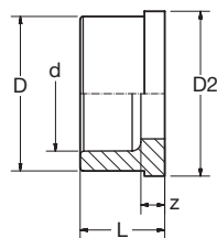
G 8060B PP-RCT Verschraubung Einlegeteil grün PP-RCT Union Insert-part green
