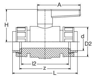
G 8852 PP-R Kugelhahn verschraubt Runddichtring-EPDM 20°C/1.0MPa grün PP-R Ball valve with union-nuts O-Ring-gasket-EPDM 20°C/1.0MPa green
