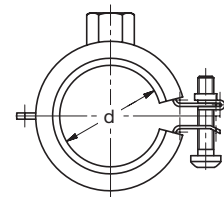
8500 Rohrschelle STANDARD mit Gummieinlage schwarz Pipe clamp STANDARD with rubber insert black
