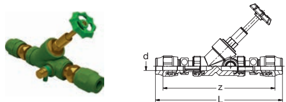
G 8650 PP-R-RG Ventil Schrägsitz mit Entleerung + Prüfstopfen verschraubt grün PP-R-Bronze Valve angle with drainage + test-plug and union-nuts green
